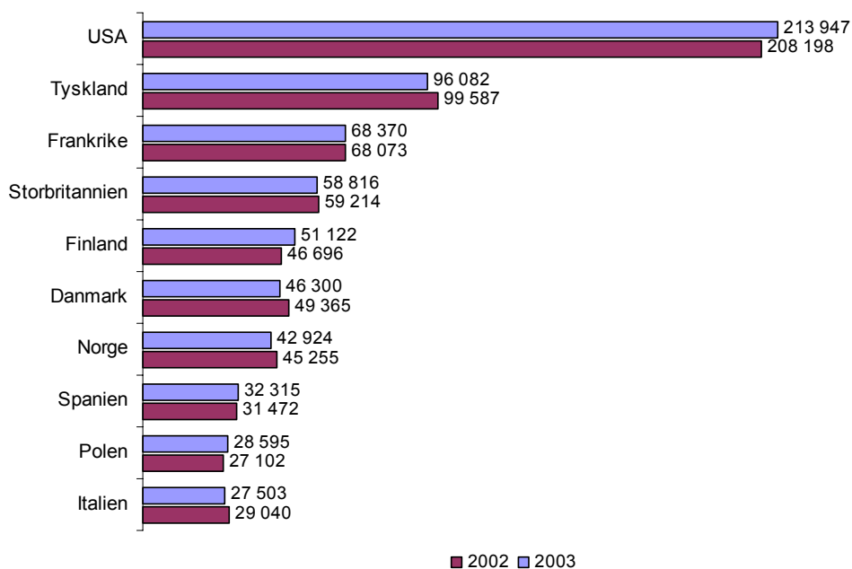
Figur 3 Länder där svenskägda koncerner med dotterbolag utomlands hade flest anställda 2003.
